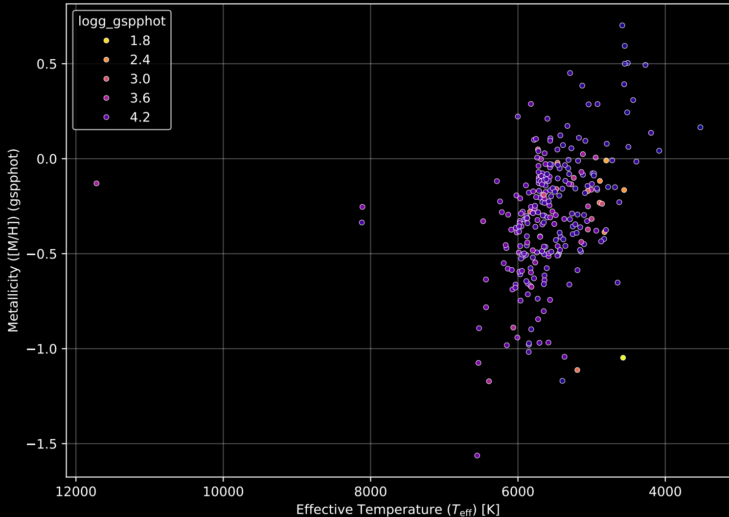
GALAH DR4 Field: [6834] Stellar Population Parameters (n= 270)
