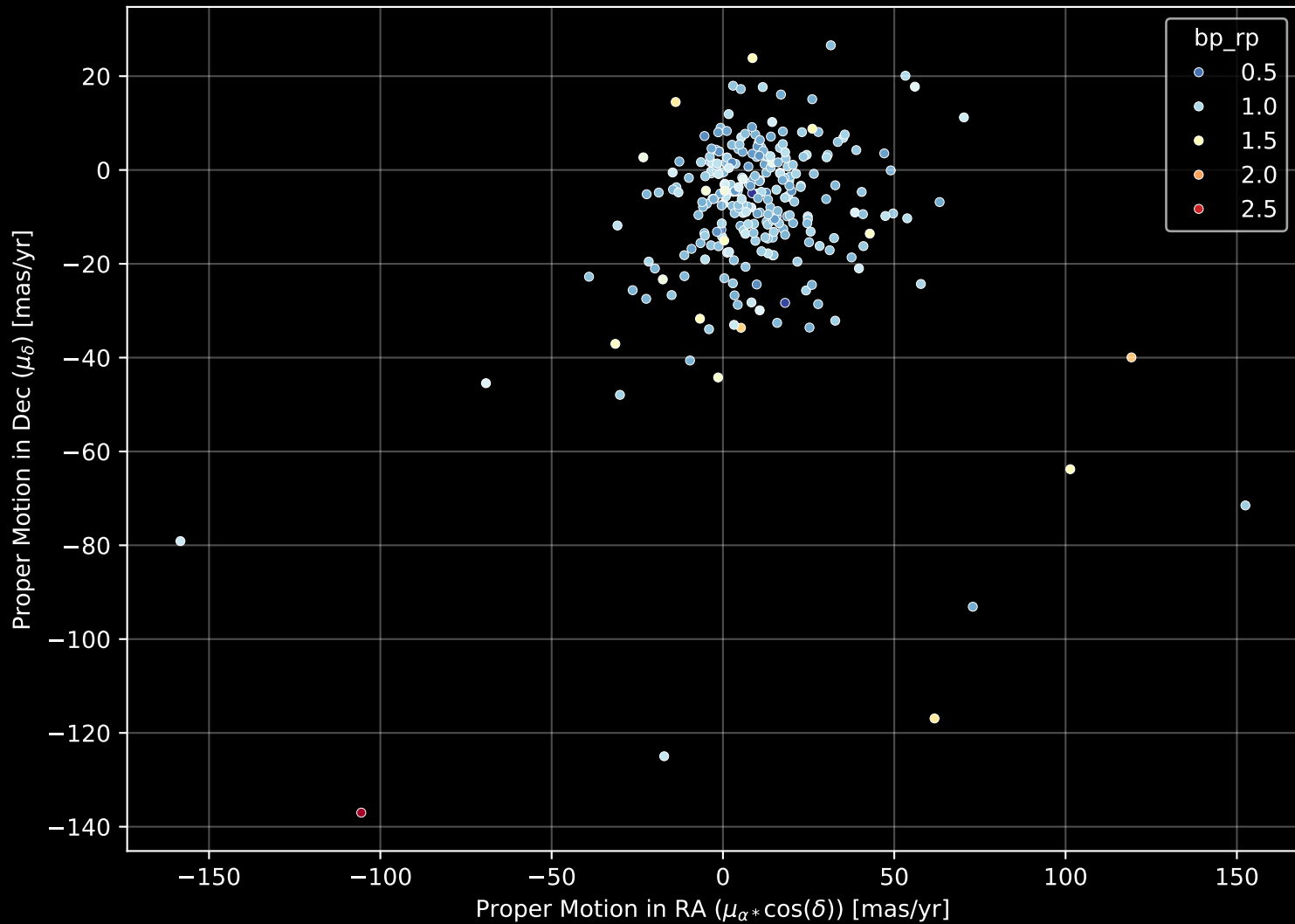
GALAH DR4 Field: [6834] Proper Motion Diagram (n= 270)
