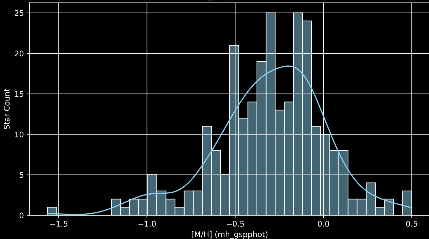
GALAH DR4 Field: [6834] [M/H] (mh_gspphot) (n= 267)
