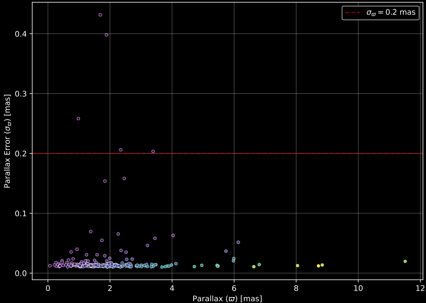
GALAH DR4 Field: [6834] Parallax Quality (n= 270)
